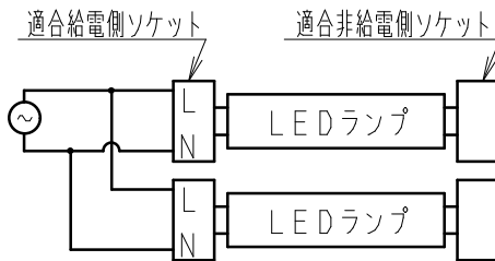
2灯用結線図
