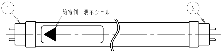
全体図 1/10
